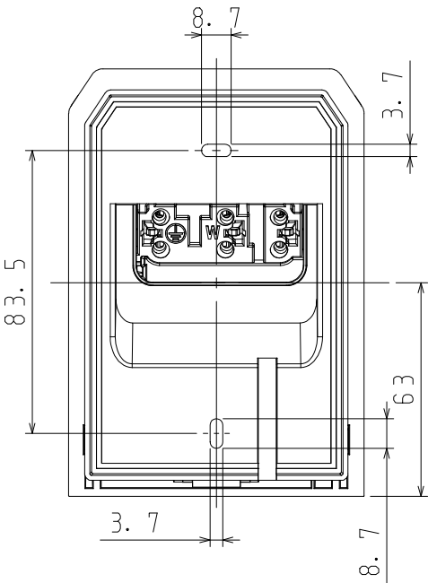
背面寸法
