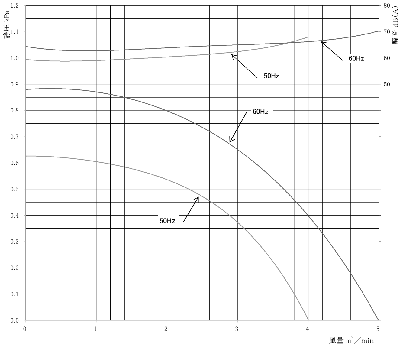
性 能 曲 線 20 °C 換 算 値
