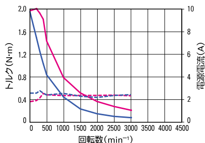
⑤ モータ型番 PBM604FXE20
