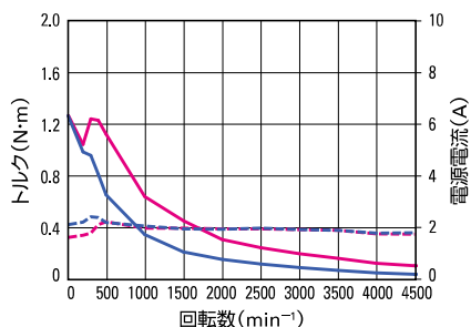
④ モータ型番 PBM603FXE20
