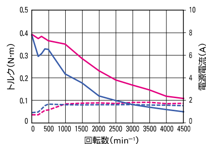
③ モータ型番 PBM423FXE20
