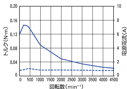
② モータ型番 PBM284FXE20
