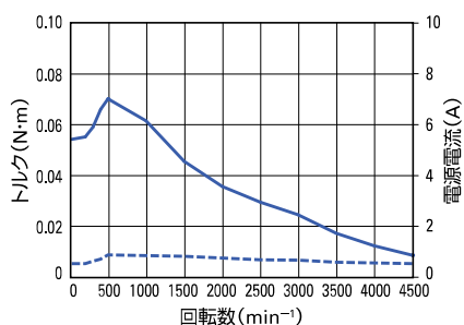
① モータ型番 PBM282FXE20
