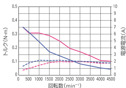
① モータ型番 PBM423DXR50
