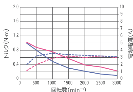
② モータ型番 PBM603DXR50
