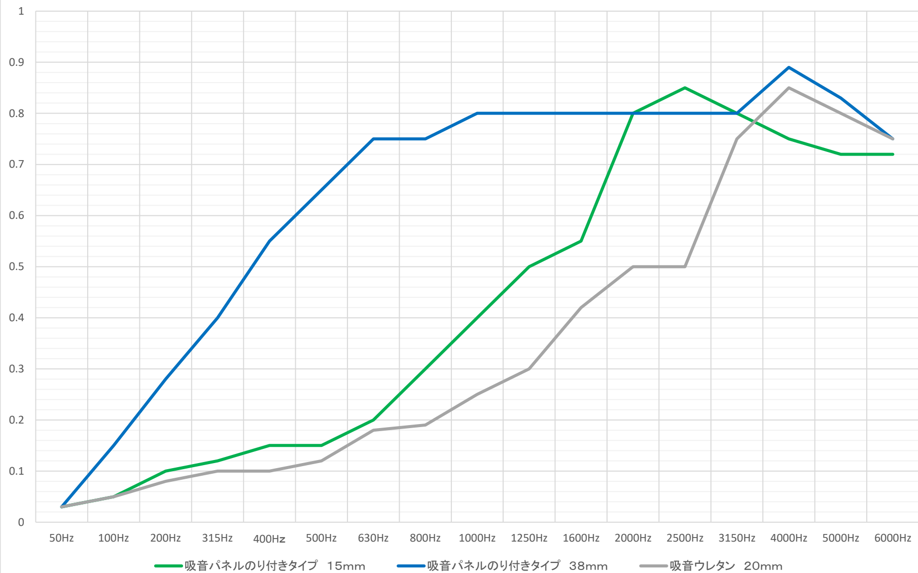
吸音率比較(垂直入射にて比較)
