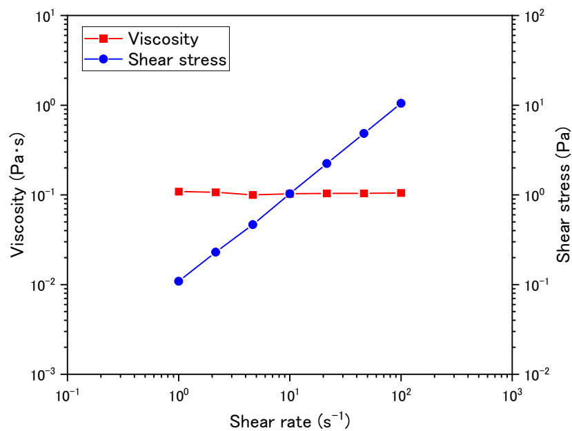
図-1 TB1373N の流動曲線
