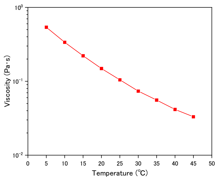
図-2 TB1373N の温度-粘度曲線
