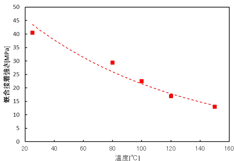
図-3 TB1373N の熱時嵌合接着強さ (ピン/カラー)
