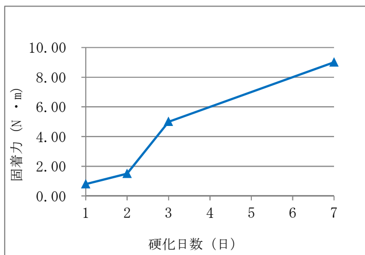
図-1 硬化速度
