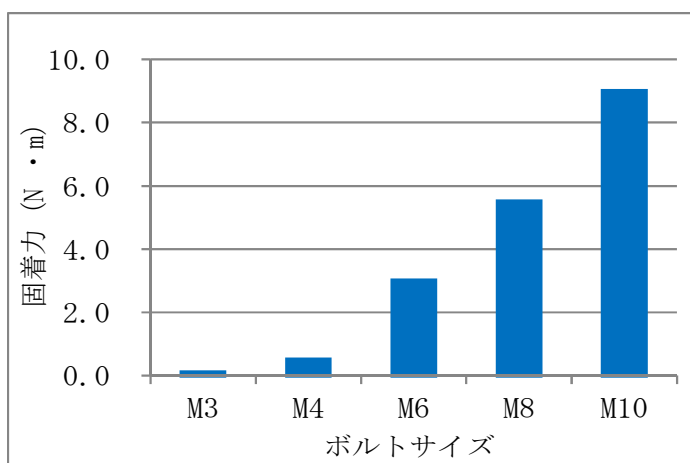
図-2 サイズ別固着力
