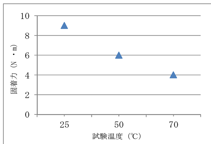
図-3 各温度下における固着力
