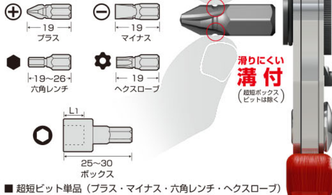
■ 超短ビット単品 (プラス・マイナス・六角レンチ・ヘクスローブ)
