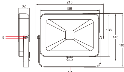
防雨型 3 芯アース付きプラグ採用
