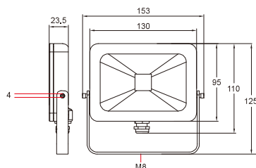
防雨型プラグ採用
