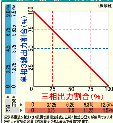
三相と単相3線の出力配分率 (概念図)
