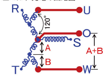
■マルチ発電の回路図
