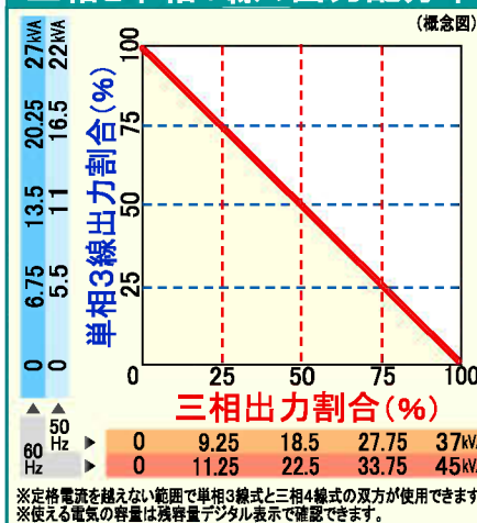
三相と単相3線の出力配分率
