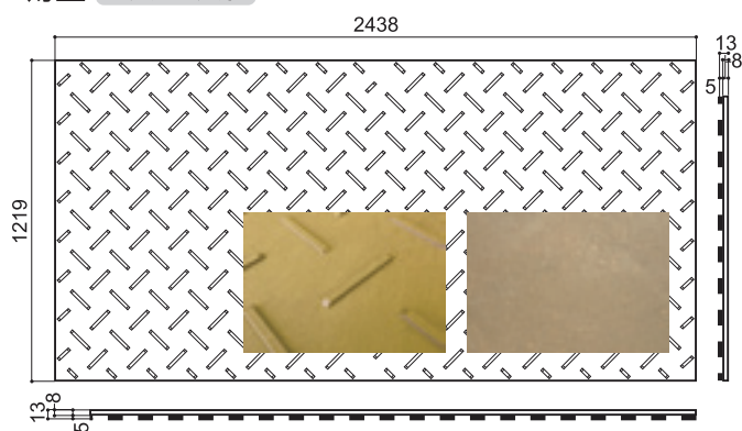
薄型 4尺×8尺判
