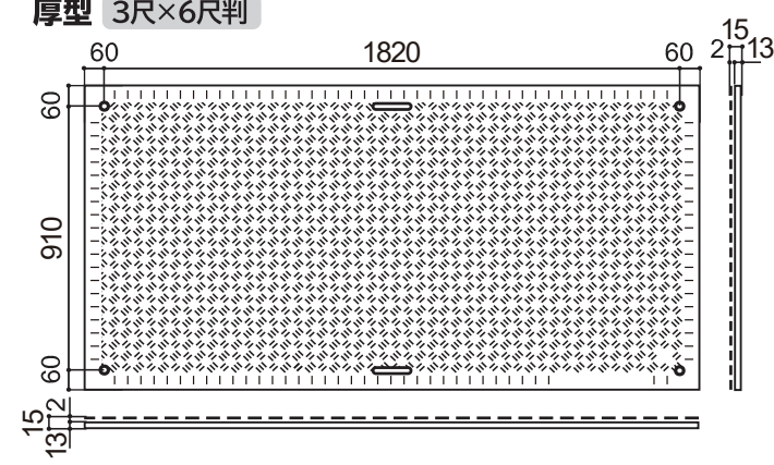
厚型 3尺×6尺判
