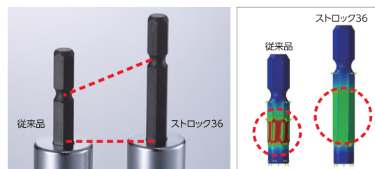
軸長さ比較
