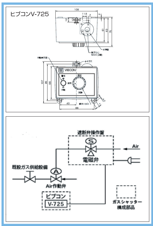
遮断弁操作盤 幅300mm×奥行160mm×高さ400mm
