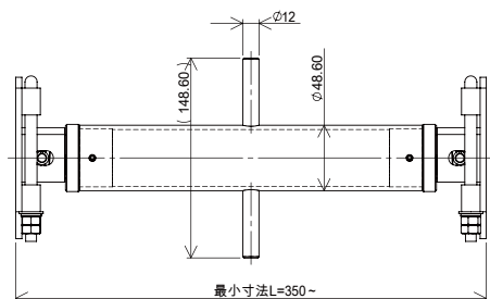
両ネジタイプ (35-55 型、50-70 型)
