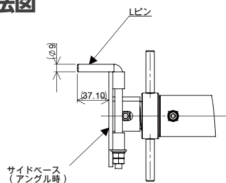
両ネジタイプ (35-55 型、50-70 型)
