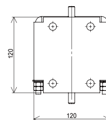
両ネジタイプ (65-100 型、95-130 型、125-160 型)
