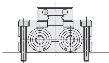
貫通穴仕様
