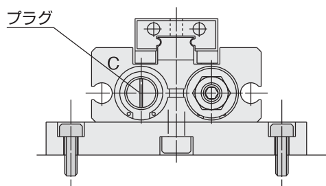
標準仕様
