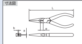
バネ部 (J100R/J115R/J150RS)
