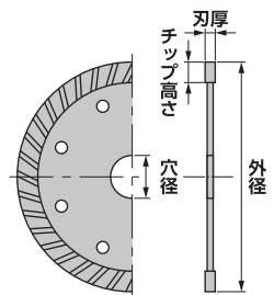
ウェーブタイプ (JCW,PCW)
