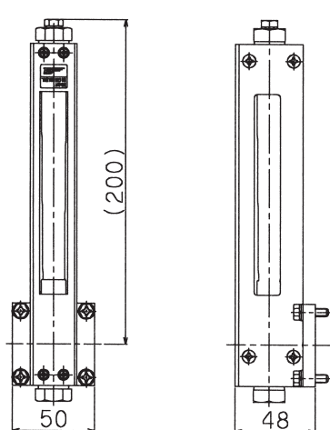
材質 (SCS14)
