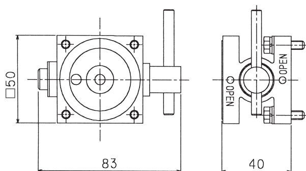
材質 (SCS14)
