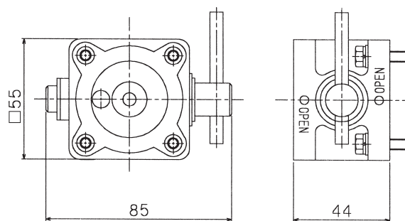
材質 (HT-PVC)
