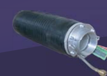
止水ボール 大流量タイプ
