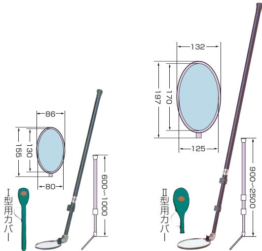
ミラーⅠ型 600～1,000mm (2段継)
