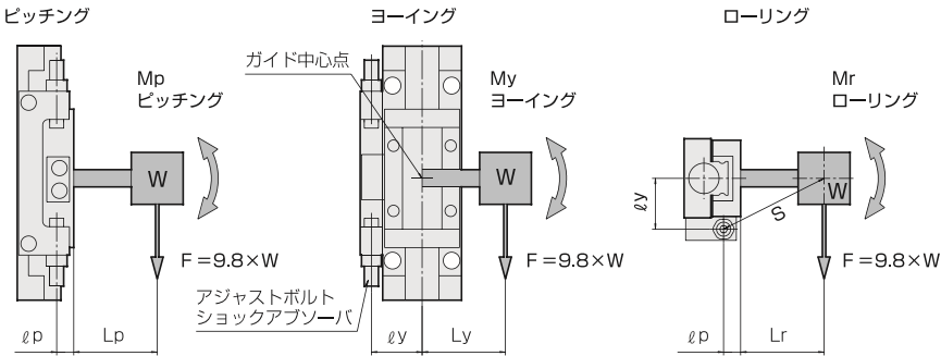
アジャストボルト、ショックアブソーバ位置寸法 単位: m
