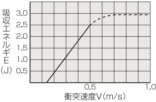
吸収エネルギーグラフ
