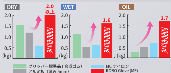
把持重量試験比較 ※当社測定代表値 UR3にて30秒把持できる重さの測定値
