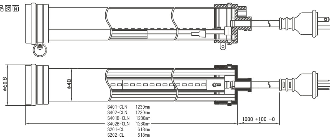
S401-CLN 100Vプラグ S401B-CLN 100Vプラグ S201-CL 100Vプラグ
