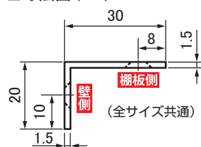
■寸法図 (mm)
