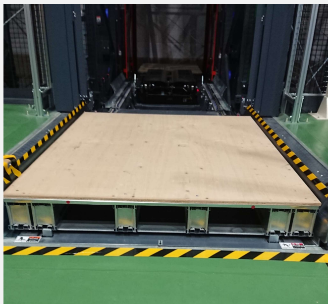
例：2,000kg積載時に撓み10mm以内
