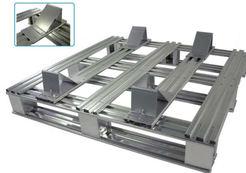
「転がり止め」を4カ所溶接
