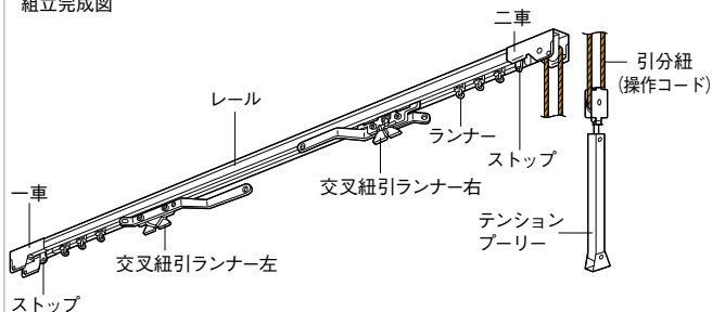
組立完成図
