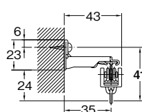
シングルブラケット付 (ブラケット幅=18mm)
