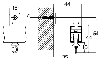
シングルブラケット付
