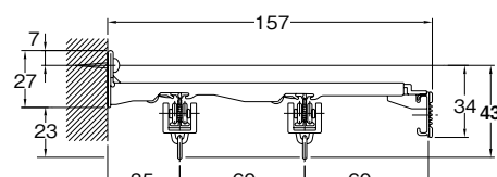
バランス用ダブルブラケット付 (ブラケット幅=18mm)
