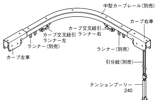
カーブ紐引部品セット組立図
