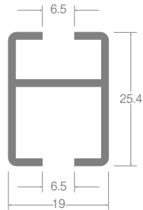
レール断面図 (単位: mm)
