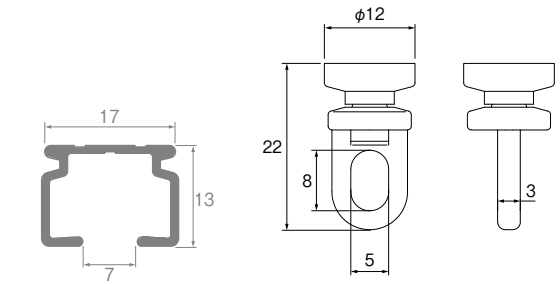
レール断面図 (単位: mm)
