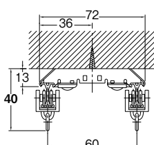
ワンタッチ天井付 ダブルブラケット付 (ブラケット幅=19mm)
