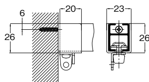
壁面ブラケットB付
