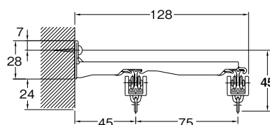
エキストラダブルブラケット付 (ブラケット幅=24mm)
