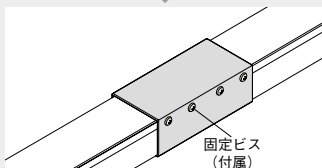
付属の 4 本の固定ビスを締めるとレールが固定されます。
