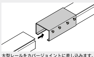
大型レールをカバージョイントに差し込みます。
