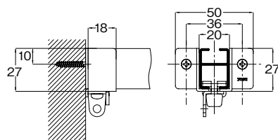
壁面ブラケットA付
