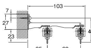
ダブルブラケット付 (ブラケット幅=18mm)
