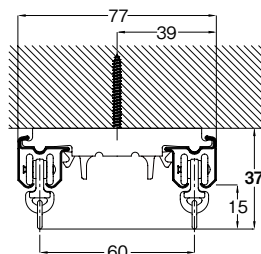
天井付ダブルブラケット付 (ブラケット幅=18mm)
