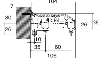
カバートップⅡセット側面図
