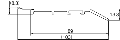
カバートップⅡ本体側面図
