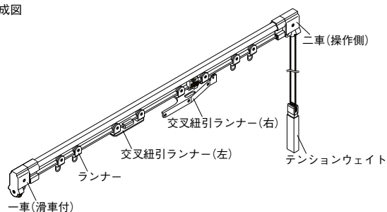
組立完成図
