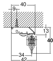
ワンタッチ天井付 シングルブラケット付 (ブラケット幅=18mm)
