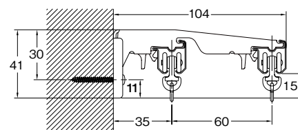
LTダブルブラケット付 (ブラケット幅=35mm)
