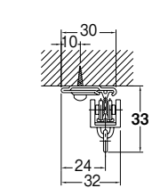
天井付シングルブラケット付 (ブラケット幅=14mm)
