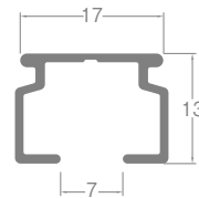
レール断面図（単位：mm）
