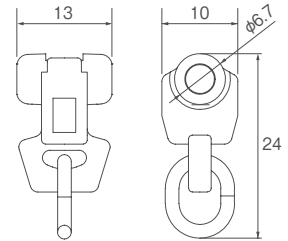
ランナー寸法図（単位：mm）
