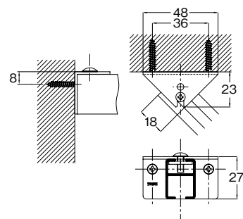
特殊壁面ブラケット付
