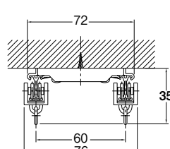
天井付ダブルブラケット付 (ブラケット幅=18mm)
