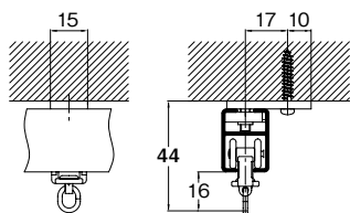
天井付シングルブラケット付
