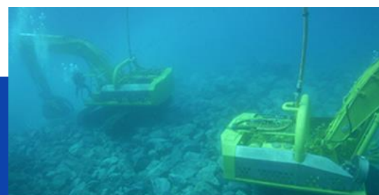
水中バックホウへの給電
