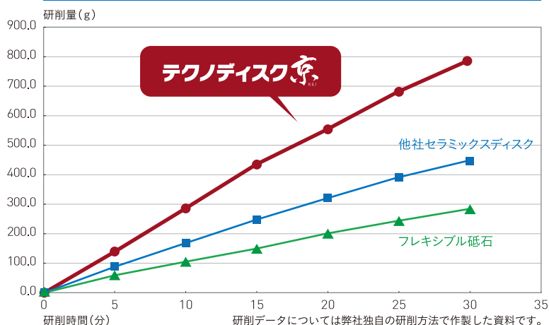
SS400材研削データ
