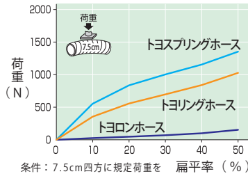
■ つぶれ強度比較（50φ）
