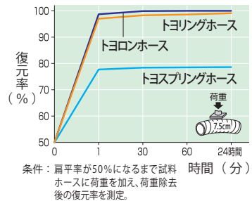
■ 復元性比較（50φ）
