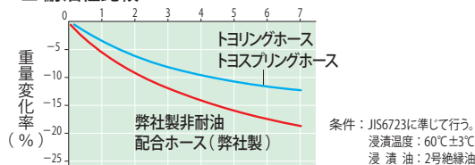
■ 耐油性比較 浸漬日数（日）
