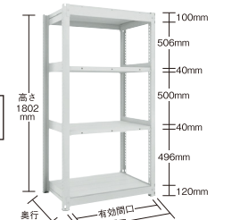
TUG60063L4 (単体型)
