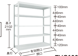
TUG60076L5 (単体型)
