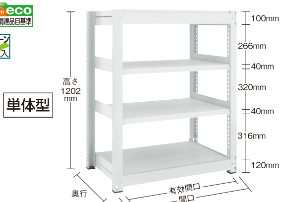
TUG45043L4 (単体型)
