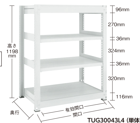
TUG30043L4 (単体型)
