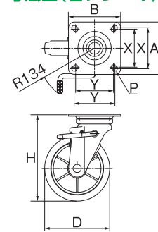
寸法図(右ブレーキ)
