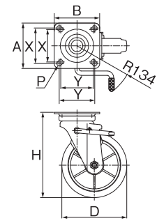
寸法図(左ブレーキ)
