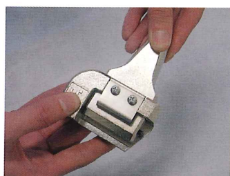
①手打ちホルダー大をセーフティグリップに上から差込みます。
