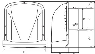
寸法図
