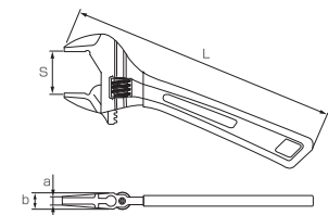
寸法図
