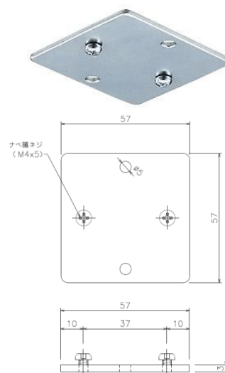
伸縮吊棒下地プレート (12Y97/15Y97/19Y97)
