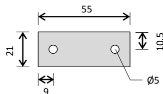
大型伸縮吊棒・天井付面寸法図
