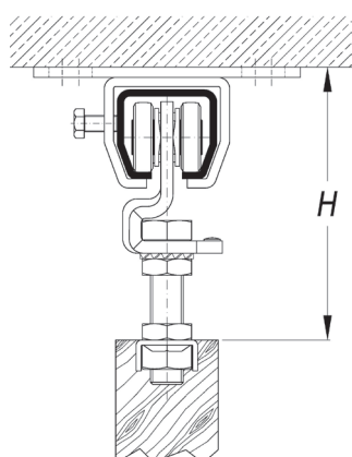
天井受一連金具と滑車(スライドドア用)
