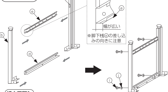
(b) 脚(③アジャスター付)…4本
