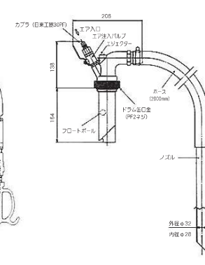
図2 APDQ (吸入専用)
