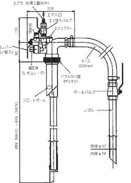
図3 APDX (吸入・吐出両用)
