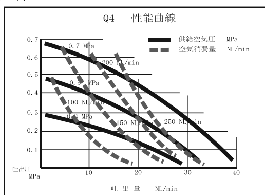
DF4D-20(G/AS)
