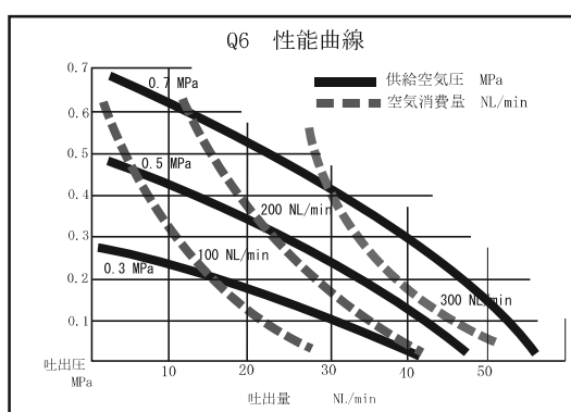
DF6D-20(G/AS)
