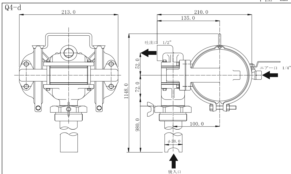
DF4D-20(G/AS)
