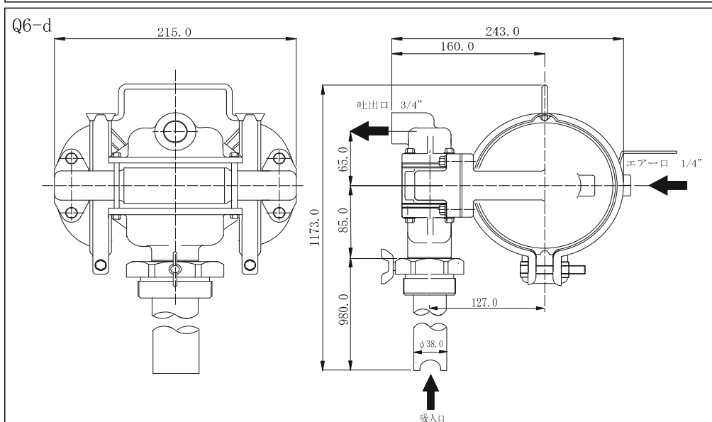
DF6D-20(G/AS)
