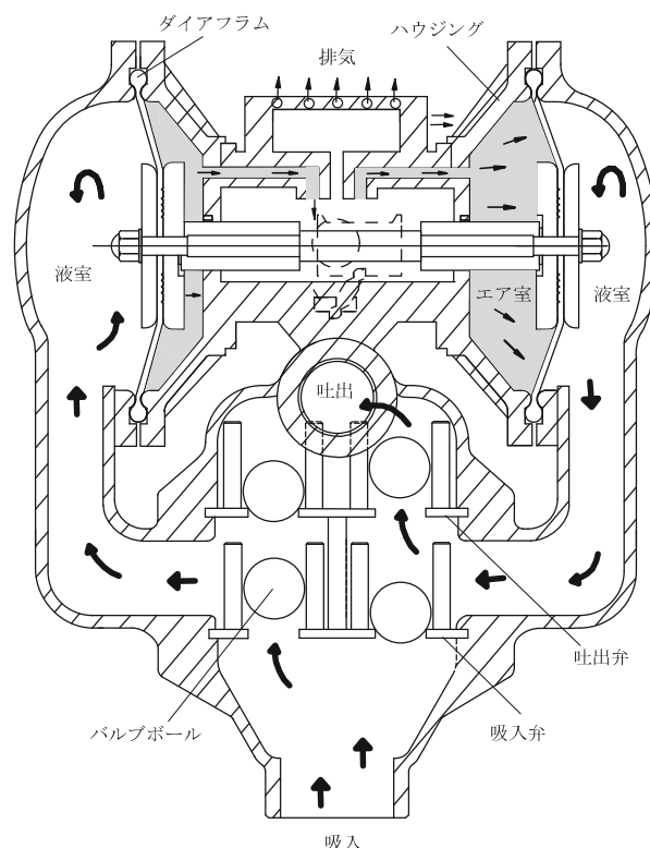
DF4D-20(G/AS)
