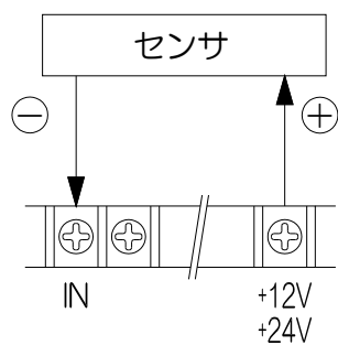
直流2線式センサ (4~20mA)
