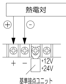
熱電対入力オプション (J・K型)
