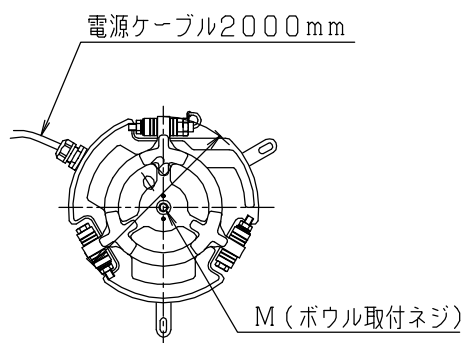
DMS-15C,20C
