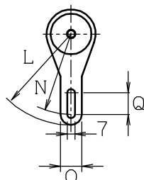
防振ゴム座
