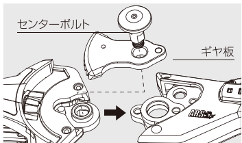
④センターボルトとギヤ板を外し、連結部を取り外します。
