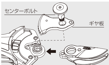
⑤EP-720の上刃下刃を入れてセンターボルトとギヤ板を取り付けます。
