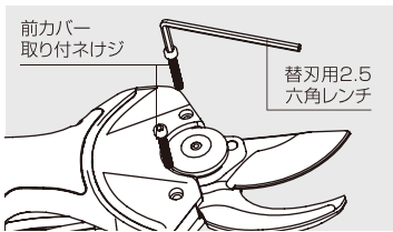
⑥本体ケースに前カバーを取り付けて前カバー取り付けネジを締めます。
