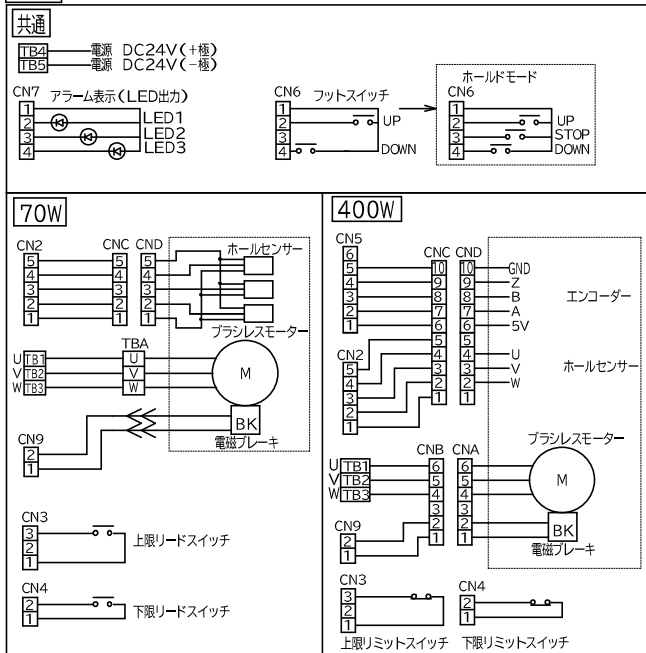
結線図
