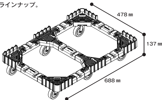
【75L オリコン用】(有効内寸:654×444 mm)
