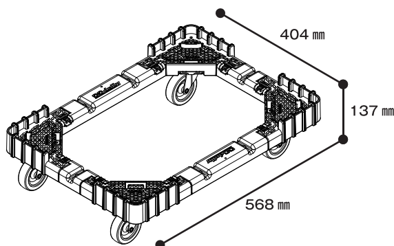
【50L オリコン用】(有効内寸:534×370 mm)
