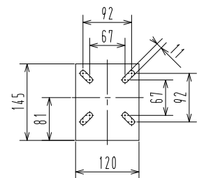
自在車用キャスター板詳細
