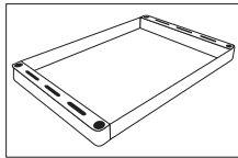
棚板 3枚 (643) 2枚 (643P) 600×406×45
