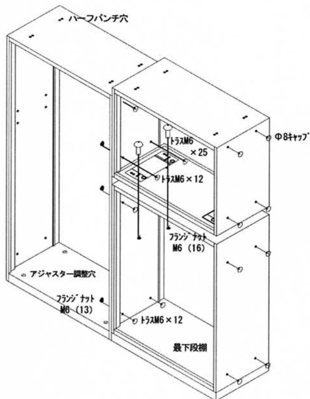
本体と本体の連結
