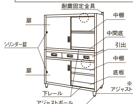
保管庫・二段式（アジャスト付）
