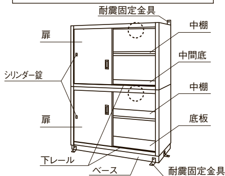
保管庫・二段式（ベース付）
