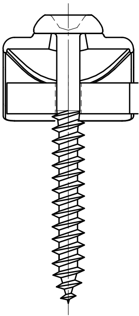
A-A断面
