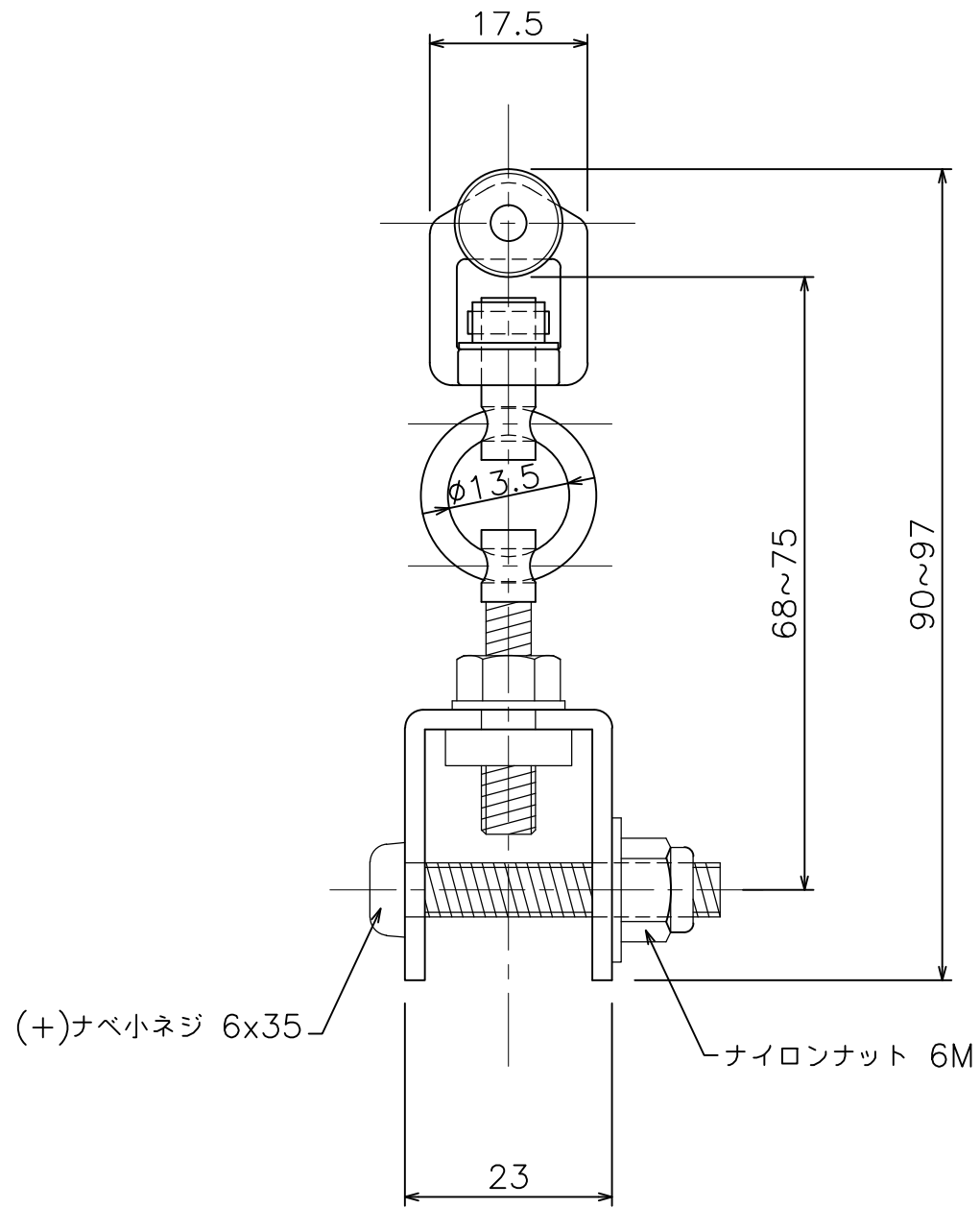
D30 間仕切用ランナー (12T28)
