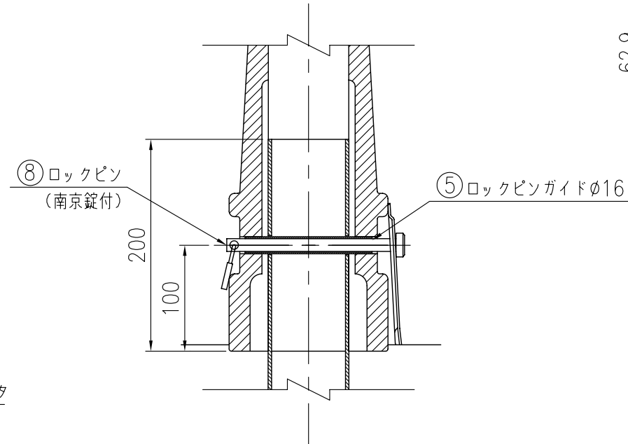
下部断面詳細図
